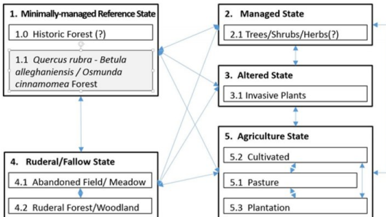
Figure 5. STM_144AY037_Moist_Dense_Till_Upland
